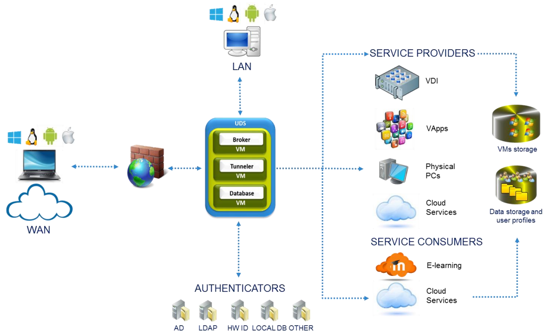
Arquitectura del software UDS Enterprise
